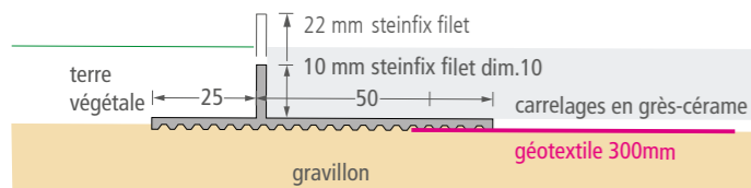
steinfix filet / steinfix filet dim. 10
